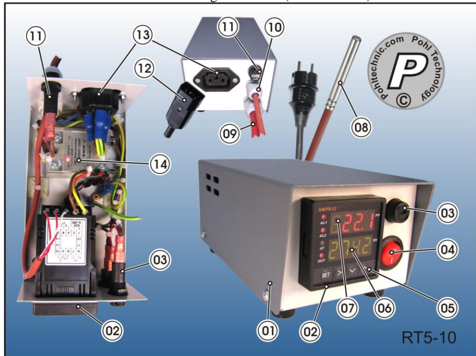
Gesamtansicht Regler RT5-xx (Abb. Ähnlich)
