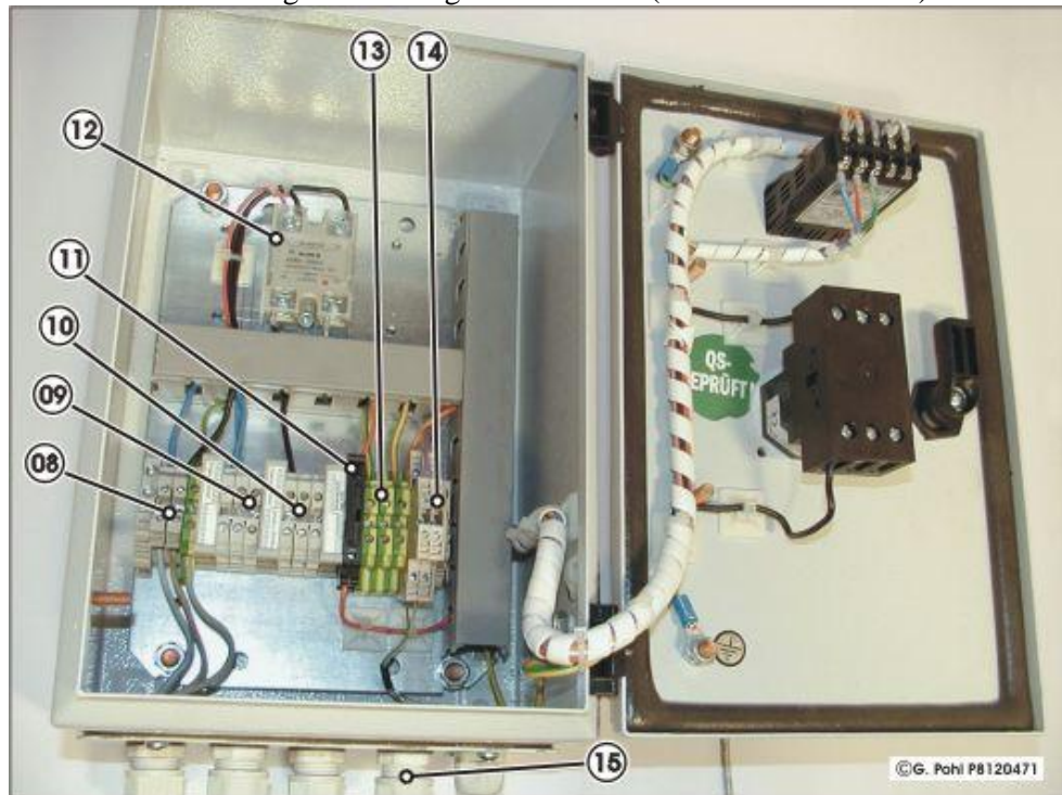
Verdrahtungsansicht Regler RT10-SSR (Modell ohne Kühler)
