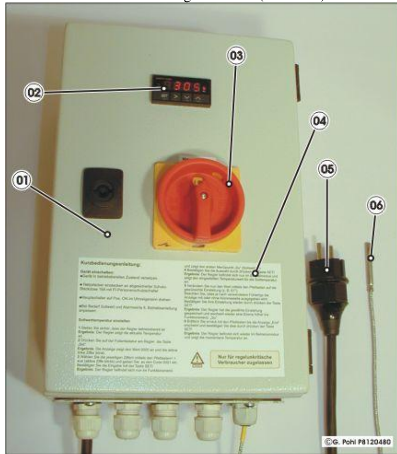
Gesamtansicht Regler RT3-13 (Abb ähnl.)
