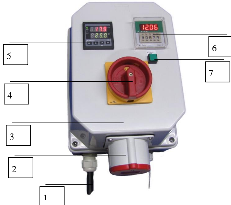
Gesamtansicht Regler RT2-51 – (Beispielhafte Abb)
