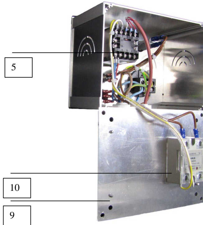
Verdrahtungsansicht Regler RT4-44
