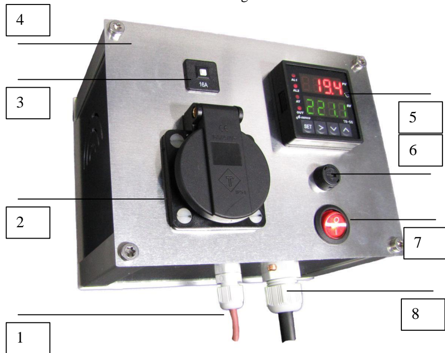
Gesamtansicht Regler RT4-44
