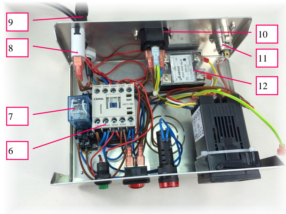
Gesamtansicht Regler RT5-194
