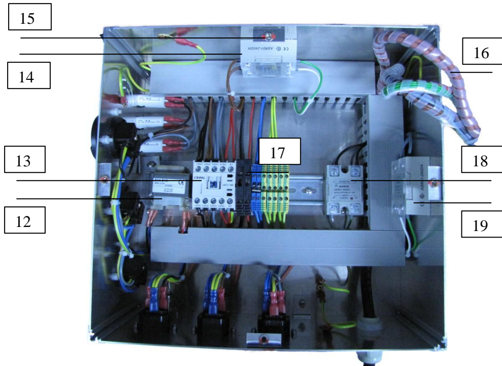
Verdrahtungsansicht Regler RT4-28
