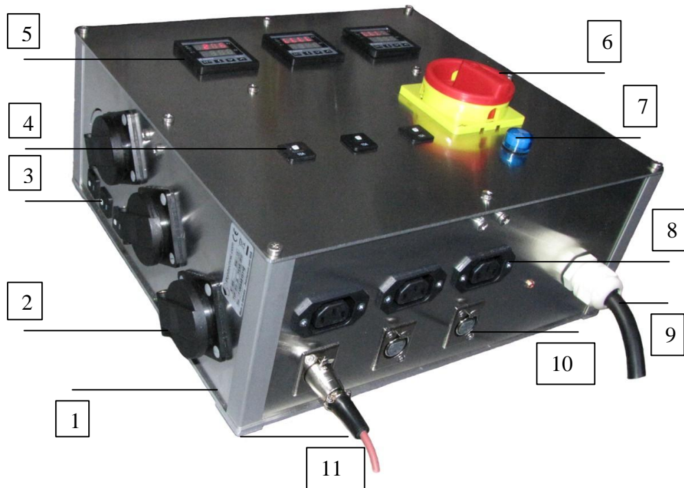
Gesamtansicht Regler RT4-28 – (Beispielhafte Abb)
