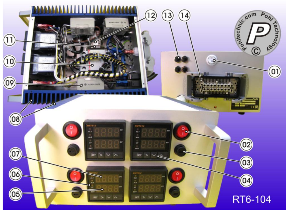
Gesamtansicht Regler RT6-104
